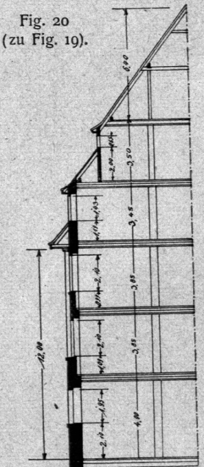
Querschnitt.
