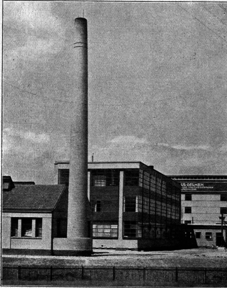
Teilansicht der Schuhfabrik Faguswerke in Alfeld 2) . Arch.: H. Gropius-Berlin.
