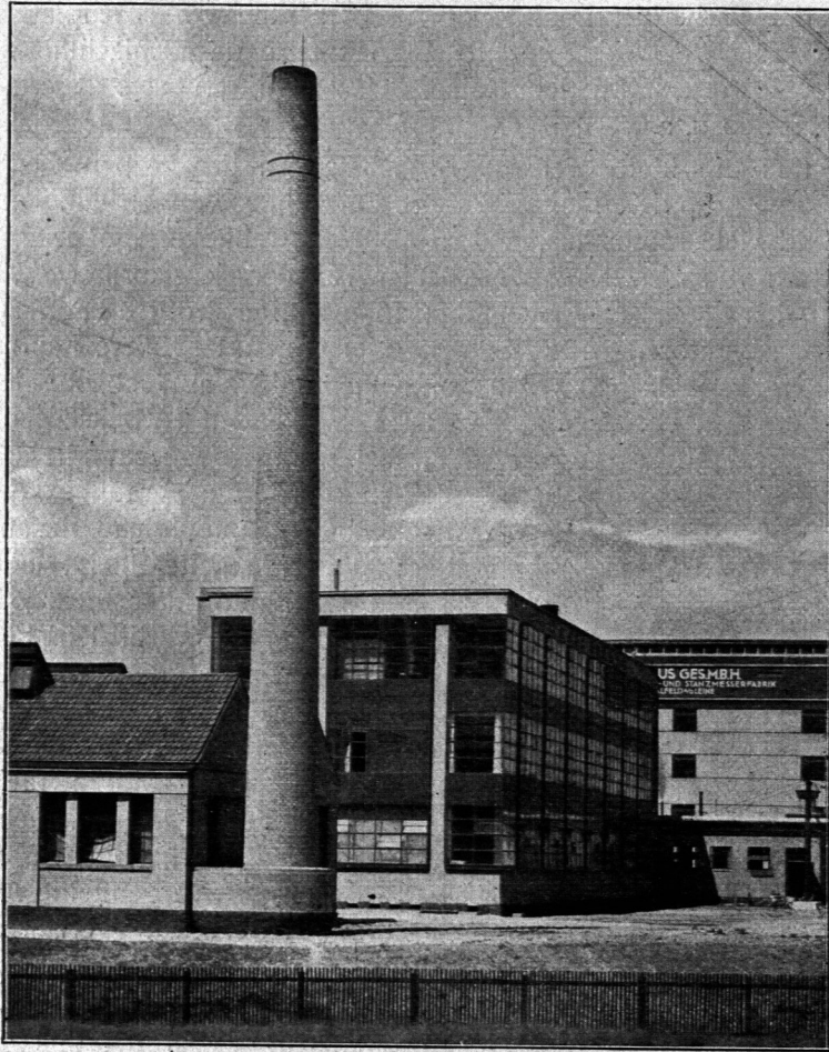
Teilansicht der Schuhfabrik Faguswerke in Alfeld 3) . Arch.: H. Gropius -Berlin.
