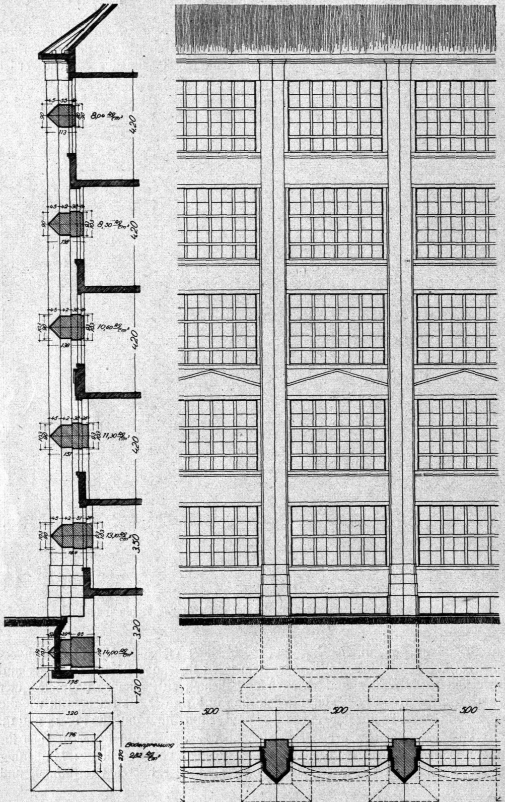
Schnitt und Anficht.
