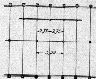
Schema für die Stützen- und Pfeilerstellung; zwei Pfeiler — eine Stütze.
