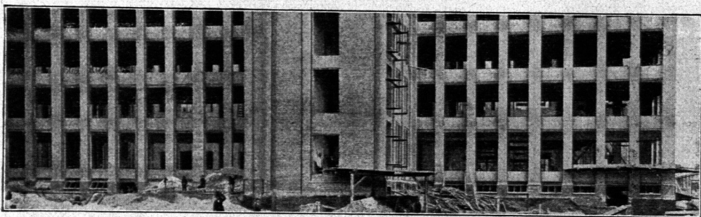
Geschossbau mit enger (2,75 m) Pfeilerstellung; die breiteren Pfeiler enthalten Rauchröhren.
