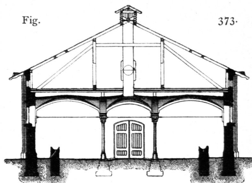
Fig. 373. Markthalle C und D auf dem Schlacht- und Viehhof zu München 163) .
