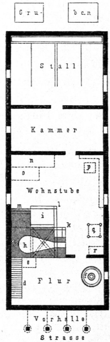
Neueres Bauernhaus. 1/200 n. Gr.
