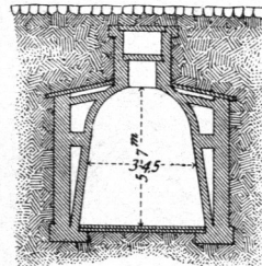
Silos. — 1/300 n. Gr.
