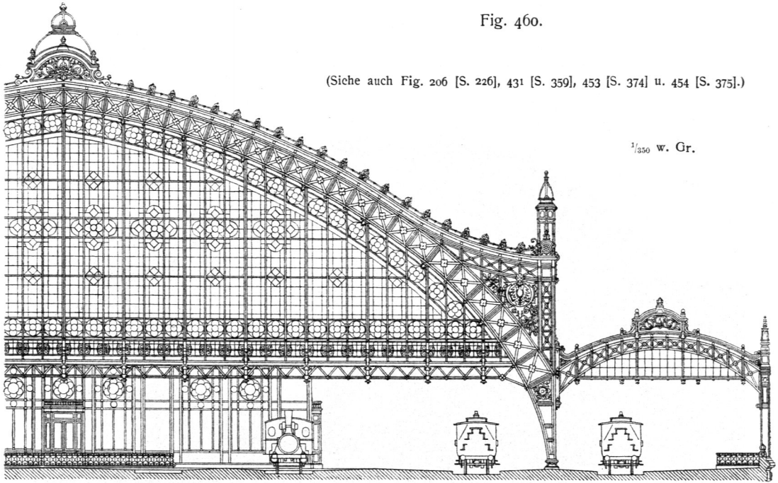
Endabfluß der Bahnsteighallen auf dem Hauptbahnhof zu Cöln 312) .
