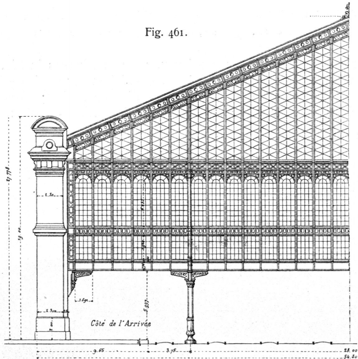
Endabfluß der Bahnsteighalle auf dem Bahnhof der Orléans-Eisenbahn zu Paris 313) .
