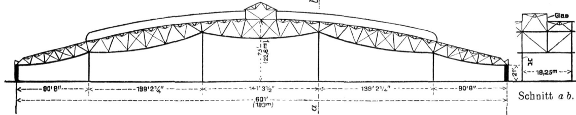
Bahnsteighalle auf dem Hauptbahnhof zu Boston 286).
