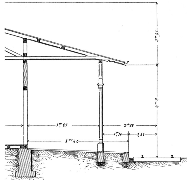
Querschnitt.
