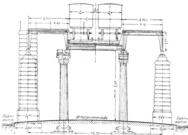
Querschnitt.
