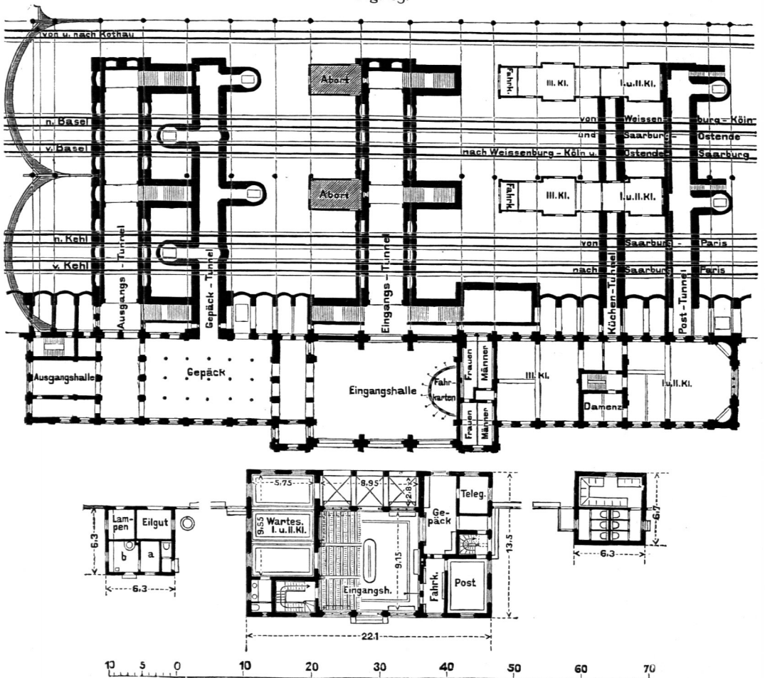
Grundriffe 64) .
