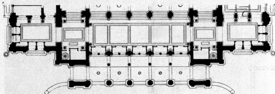
Vom Opernhaus in Wien. — 1/600 n. Gr.
