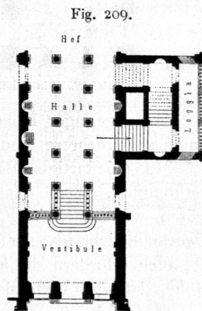
Vom Palais Brignole in Genua. \frac{1}{500} n. Gr.
