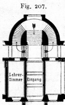
Vom Gewerbe-Vereinshaus in Mainz. — \frac{1}{400} n. Gr.
