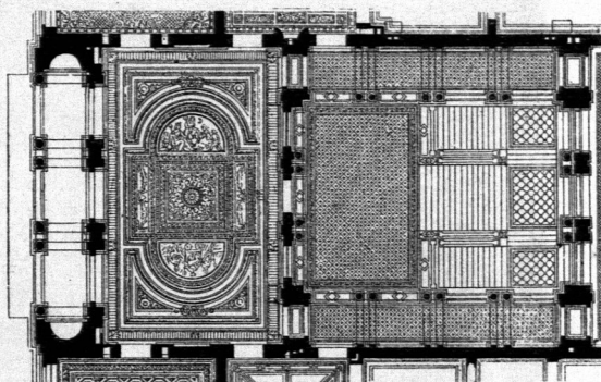
Vom Palais v. Kronenberg 96) in Warschau. — 1/420 n. Gr.
