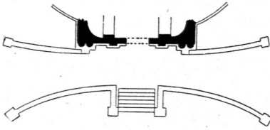
Vom Lipfius' schen Entwurf für das deutsche Reichstags-Gebäude. — 1/1000 n. Gr.
