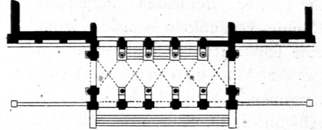
Vom alten Hoftheater zu Dresden. — 1/600 n. Gr.
