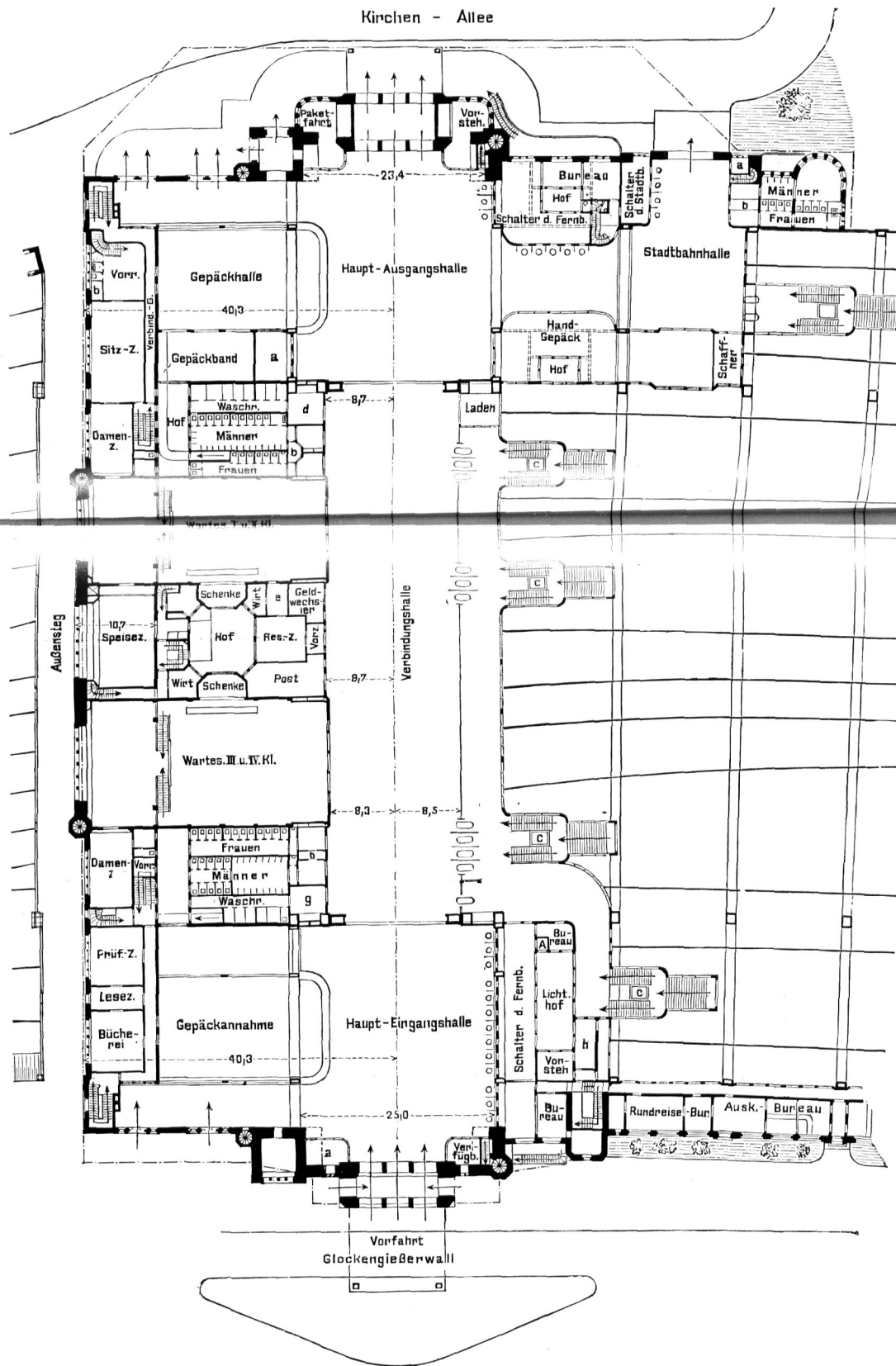
Grundriß des Erdgeschosses. — 1/600 w. Gr.
