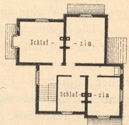
Obergeschoss.
