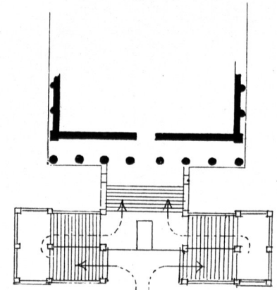
Von der National-Galerie zu Berlin. — 1/900 n. Gr. (Nach: Berlin und seine Bauten, Berlin 1877.)
