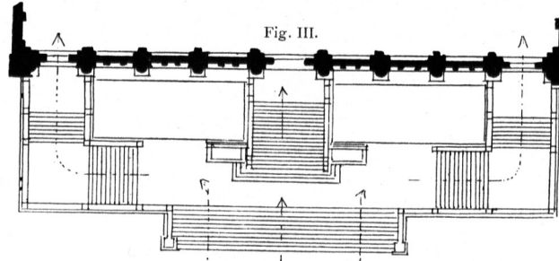
Vom Palais de justice in Paris. — 1/715 n. Gr. (Nach: Narjoux, F. Le palais de justice, Paris 1880.)
