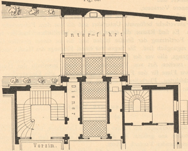
Von einem herrschaftlichen Wohnhause zu Leipzig, Karl Tauchnitz-Straße 35 71) . Arch.: Rofsbach.
