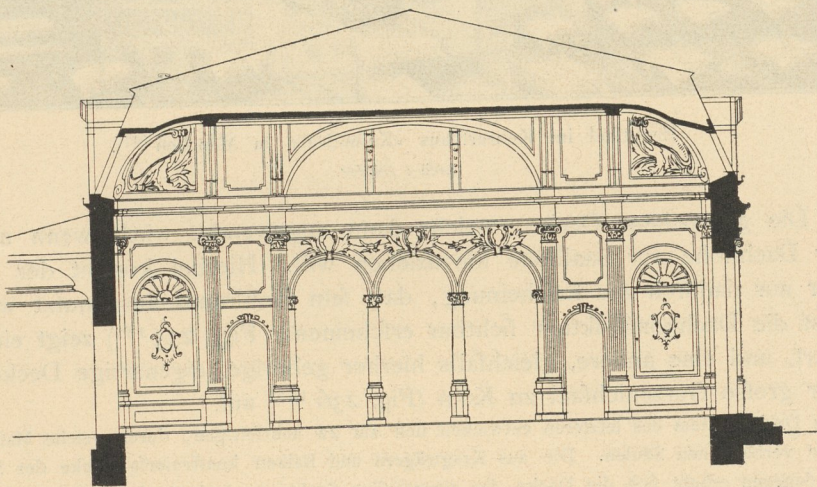
Querschnitt 160).
