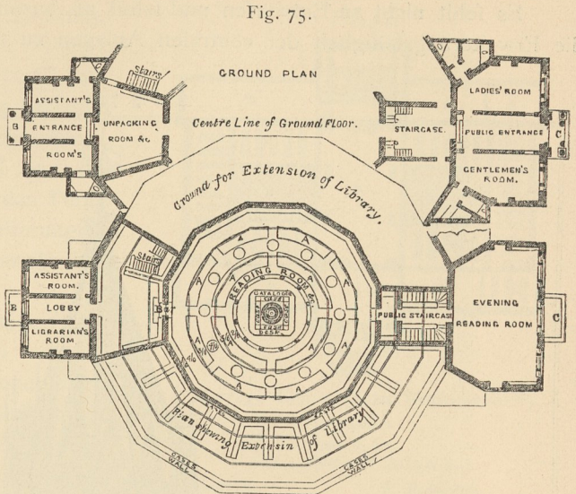
Wyatt Papworth's Entwurf für eine Bibliothek 71) . Obergeschloß.
