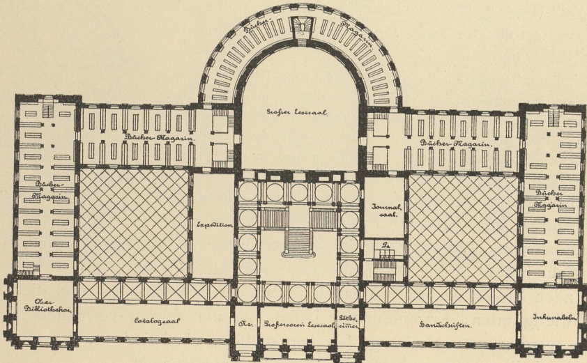
Universitäts-Bibliothek zu Leipzig. — I. Obergefchofs 67) .
