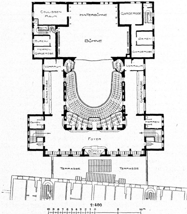
Grundriss des Erdgeschosses.
