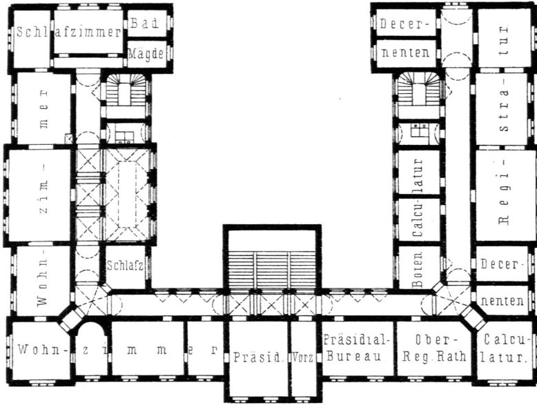
I. Obergefchofs.
