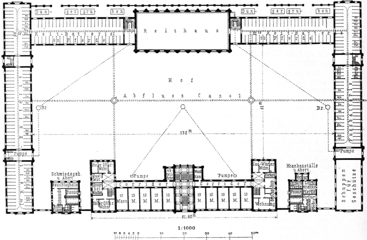
Cafernement für eine Abtheilung reitender Artillerie zu Berlin. (Erdgefhofs.)
