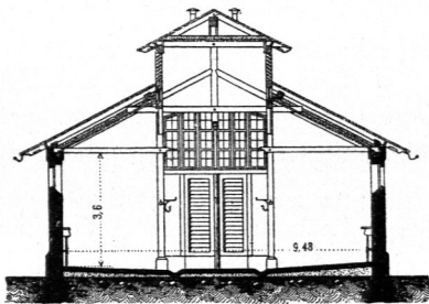
Oesterreichische Stallung älterer Construotion.
