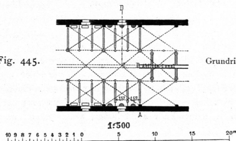
Stallung einer preussischen Artillerie-Caserne.
