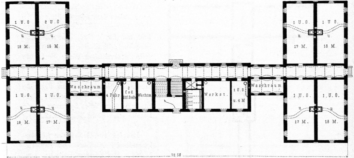
Mannschafts-Wohngebäude für 3 Escadronen. — Erdgechofs 517) .
