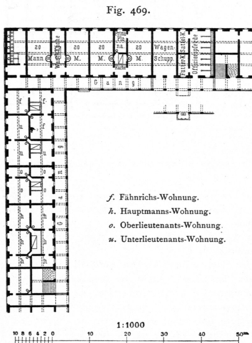
Älteres System österreichischer Infanterie-Cafernen 506 ).
