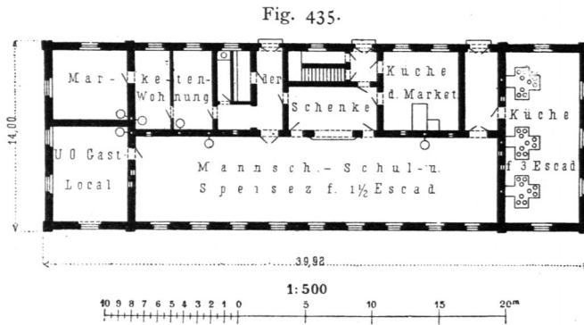
Marketenderei- und Küchengebäude einer österreichischen Cavallerie-Regiments-Caserne 482) .
