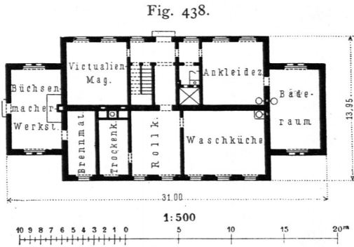
Bade- und Waschküchengebäude einer österreichischen Infanterie-Caserne 485 ).
