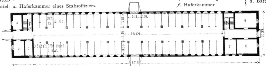
Österreichische Batterie-Stallung 495) .
