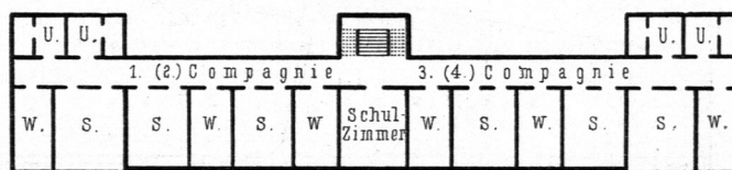
System der alt-hannoverschen Casernen (I. u. II. Obergeschoss).
