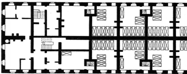
Infanterie-Caferne zu Havre 503 ).
