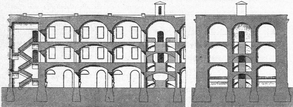
Schnitt G H H'.
