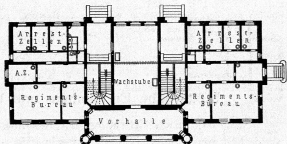
Grundriss. Wachgebäude zu Dresden — Albert-Stadt. Arch.: Rumpel.
