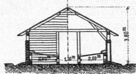
Blockwand- Flechtwerk- Baracke.
