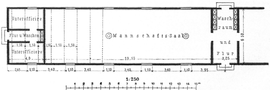
Tollet's Mannschafts-Pavillon.
