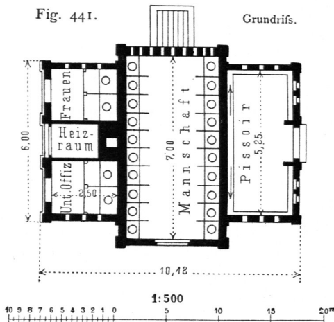
Abortgebäude für ein Bataillon in preussischen Cafernen.
