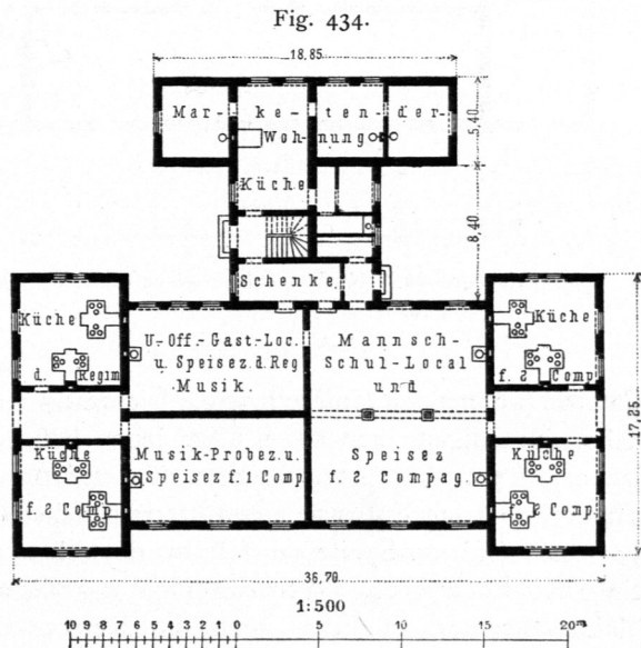
Marken-der- und Küchengebäude einer österreichischen Regiments-Caserne 480 ).
