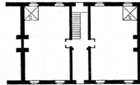
Infanterie-Caserne zu Bury 504 ).
