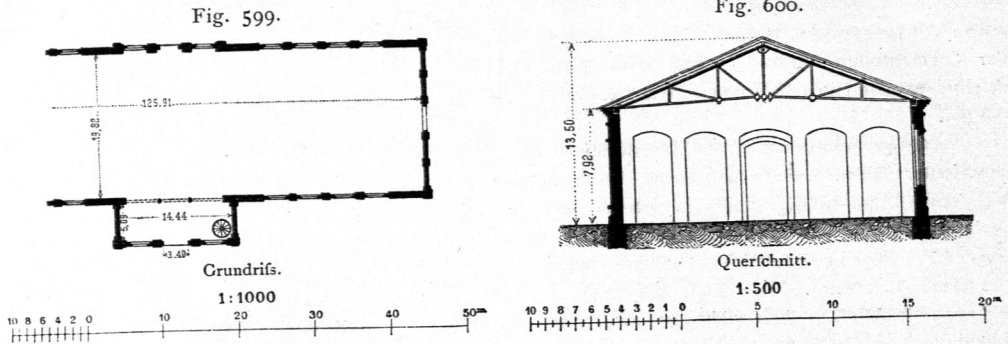
Exerzierhaus für 4 Bataillone zu Dresden.
