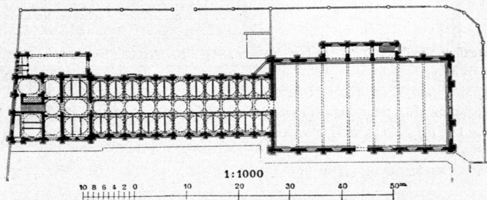
Reithaus und Stallungen der Kriegsschule zu Caffel.
