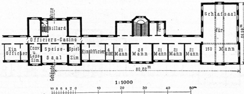
Pionier-Caferne zu Dresden. — II. Obergeschoß.
