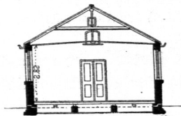
Querschnitt. — 1/250 n. Gr.
