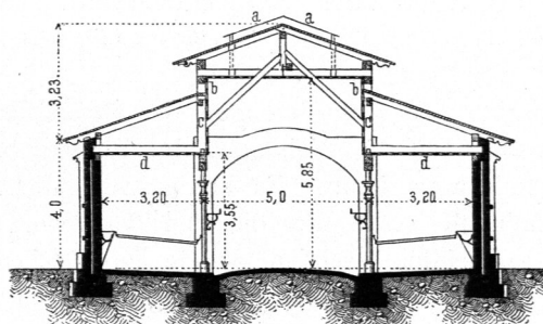
Neueres fächförmiges Stallgebäude.
