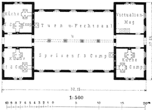
Turn-, Fechtsaal- und Küchengebäude für ein österreichisches Infanterie-Regiment 487) .
