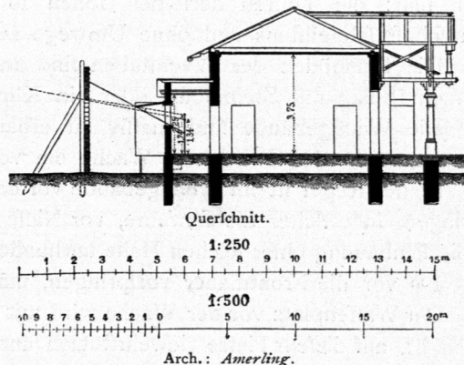
Schiefshaus mit zwei Schiefständen.
