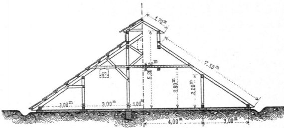
Hölzerne Stallbaracke. — \frac{1}{250} n. Gr.
