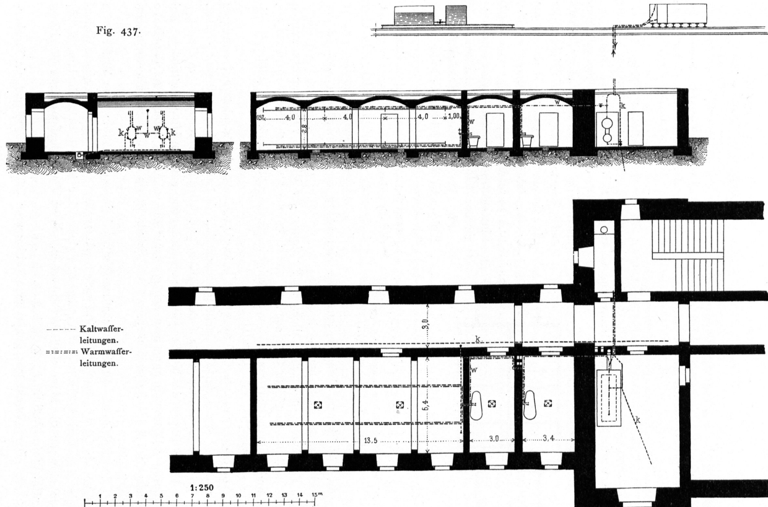
Bade-Anstalt für ein Infanterie-Regiment zu Zwickau.
