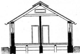
Querschnitt. — 1/250 n. Gr.
