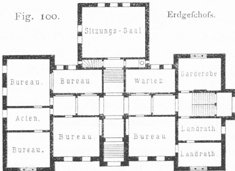
Kreisshaus zu Querfurt. — 1/500 n. Gr.
