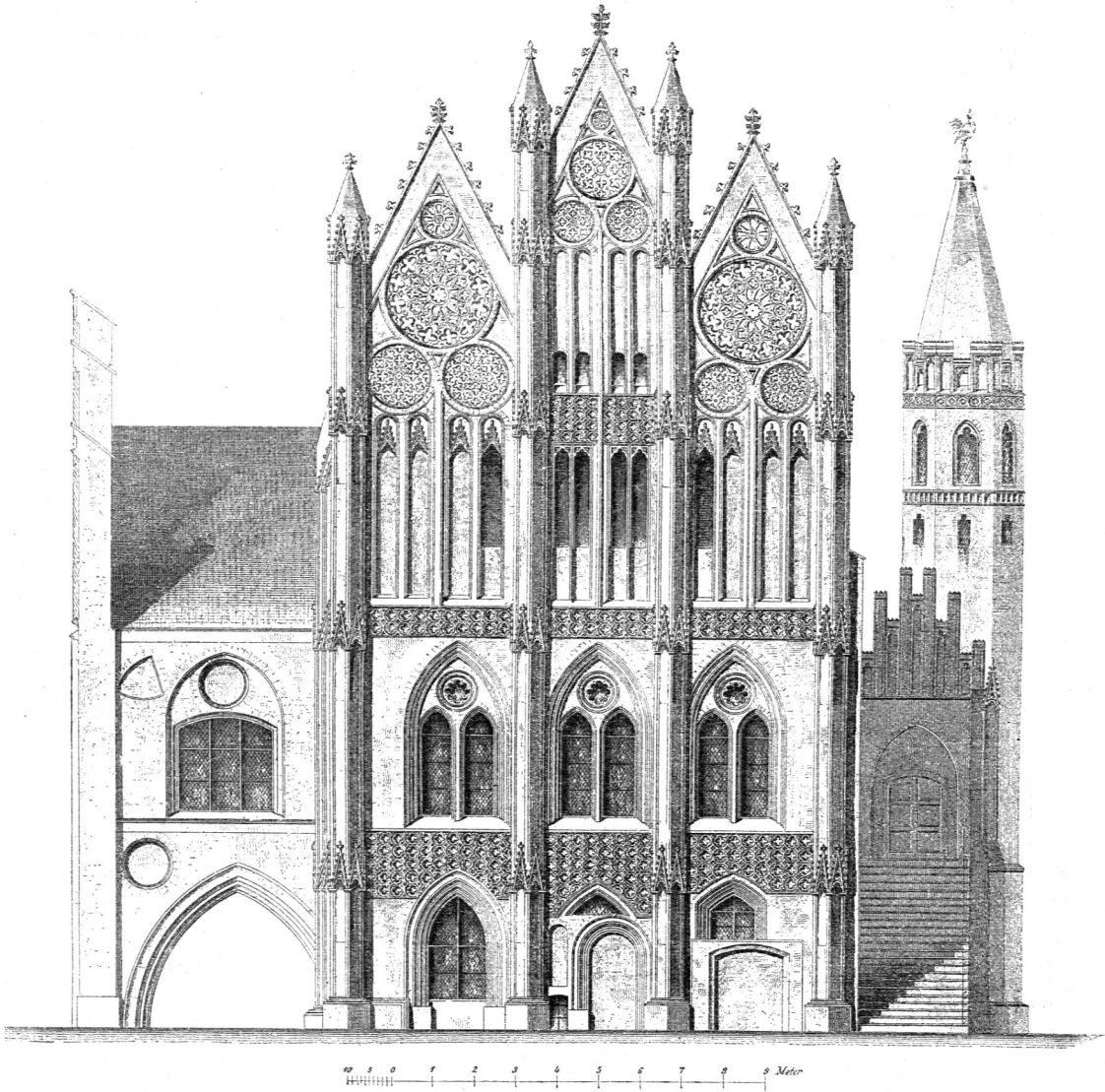
Rathhaus zu Tangermünde 21) .
