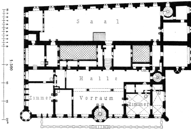
Rathhaus zu Rothenburg o. d. T. — I. Obergechofs 59) .
