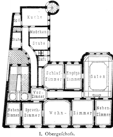
I. Obergeschoss.
