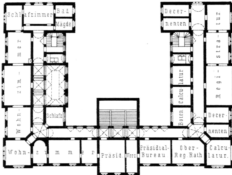
I. Obergeschoß.
