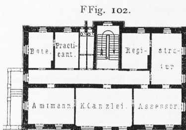
Bezirks-Amtshaus zu Pirmasens 145 ).
