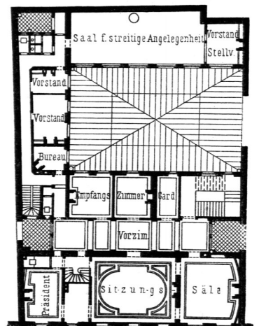
I. Obergeschoß.
