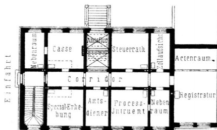
Haupt-Steueramts-Gebäude zu Potsdam 148) .
