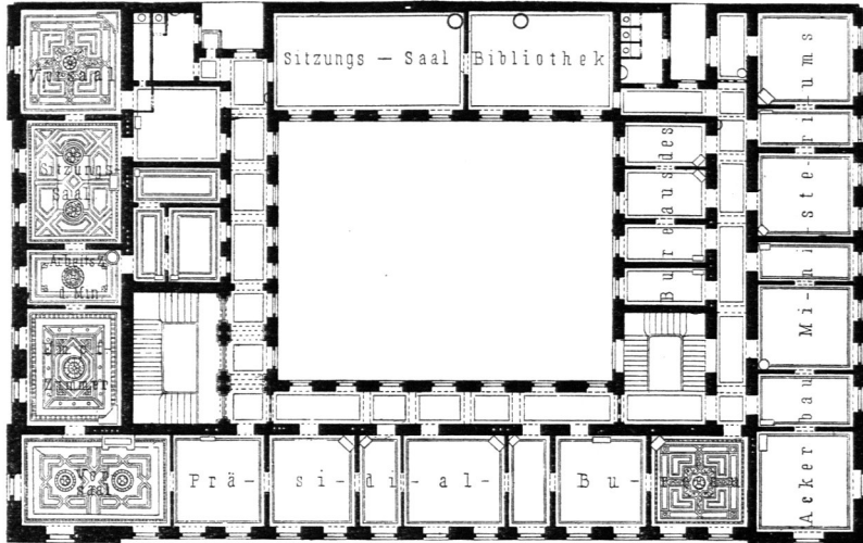
II. Obergechofs zu Fig. 70 u. 71. — \frac{1}{500} n. Gr.
