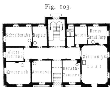
Kreis-Amtshaus zu Offenbach 146) . Erdgechofs. — 1/500 n. Gr.
