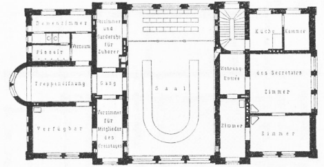
Obergeschoss.
