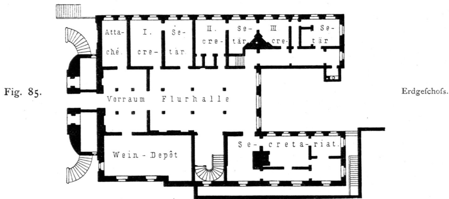
Oesterreichisches Bottschaftshaus zu Constantinopel. — 1/500 n. Gr.
