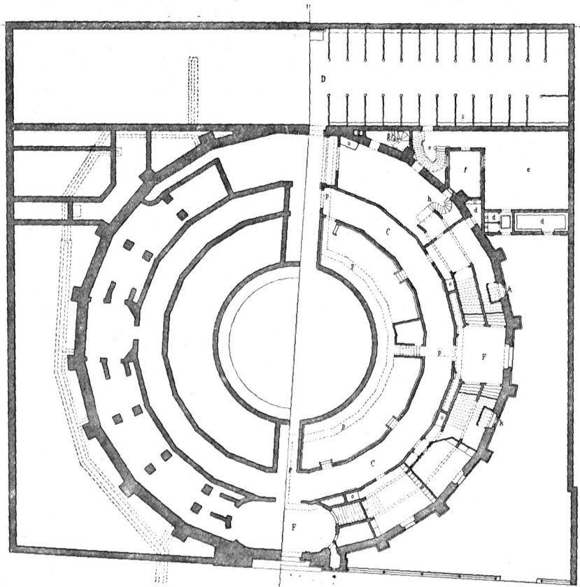
Grundriss
