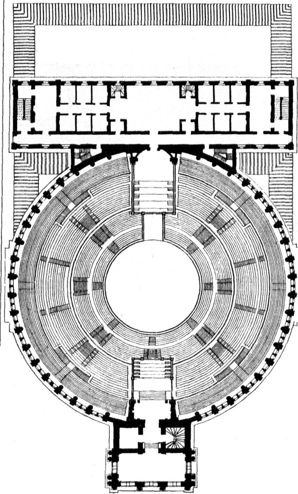
1. Obergeschoss.
