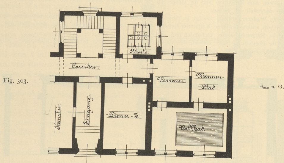
Bade-Anlage des Waifenhauses im X. Bezirk zu Wien 260 ).
