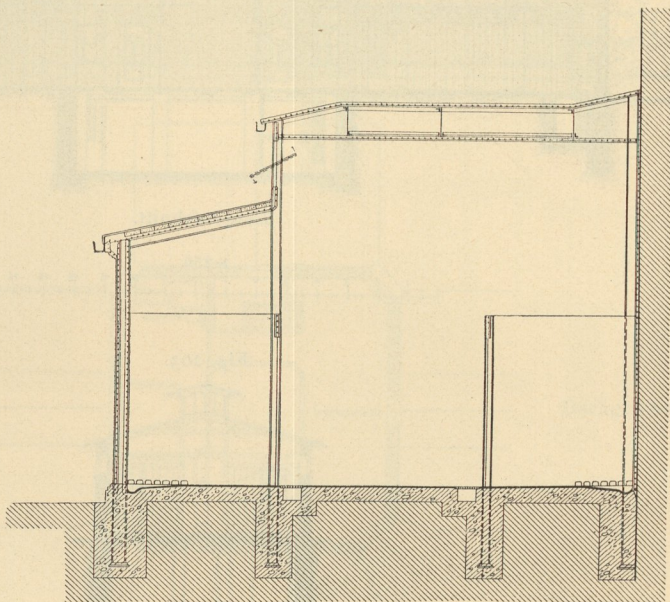
Schnitt. — 1/100 n. Gr.
