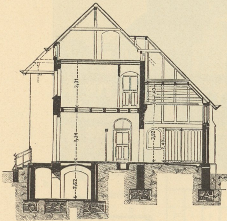
Schnitt nach AB in Fig. 209.
