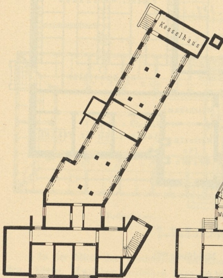
Kellergechofs.
