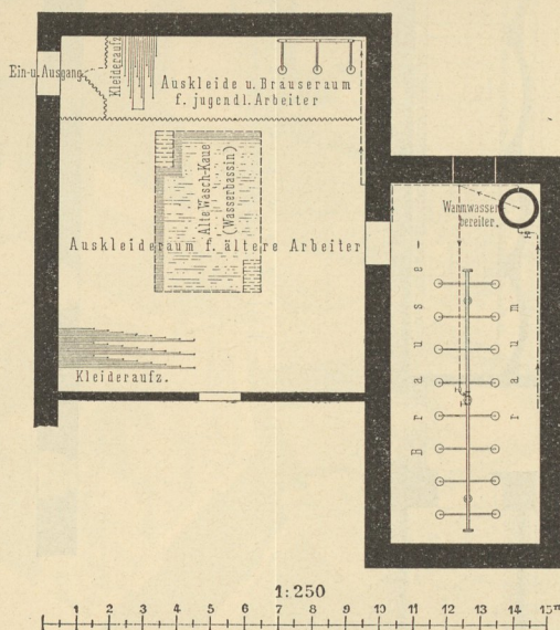
Bergwerksbad (Wafchkaue) auf Zeche »Dortfeld II« 237) .
