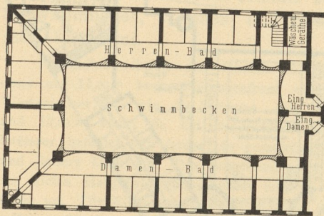
Erdgeschoß.
