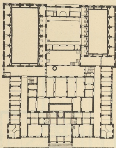
Untergechoß.
