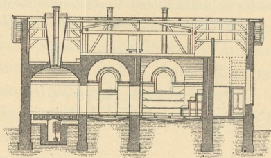
Längenschnitt.
