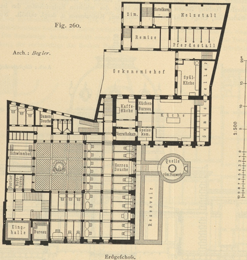
Gaft- und Badehaus »Schützenhof« zu Wiesbaden.
