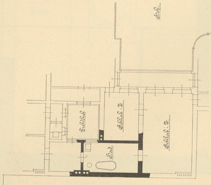
Bad im Wohn- und Geschäftshaus Friedrichstraße 240—241 zu Berlin 371), Arch.: Rossmann & Jacob.
