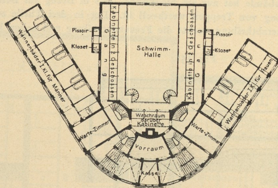
I. Obergeschloß.
