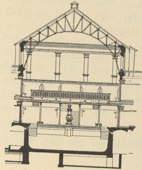
Querschnitt durch die Herren-Schwimmhalle.
