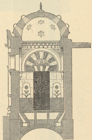
Schnitt durch den Uebergangsraum.
