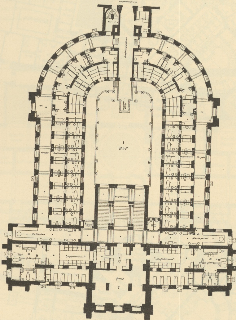
Untergeschoss. — 1/500 n. Gr.
