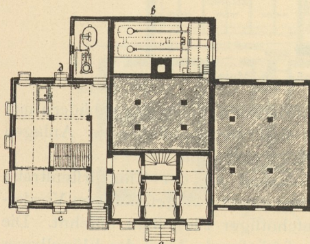
Untergechofs.
