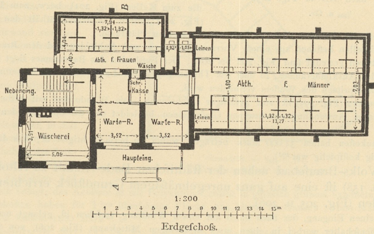
Oeffentliches Volks-Braufebad zu Breslau 222) .
