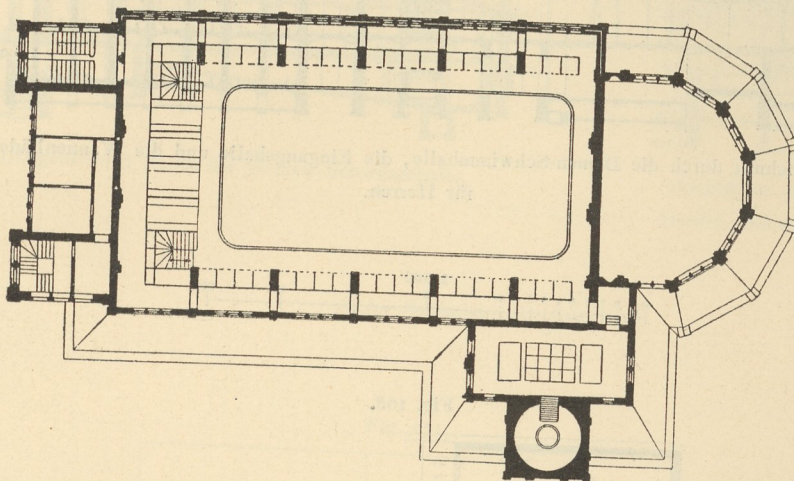
Obergeschoss.
