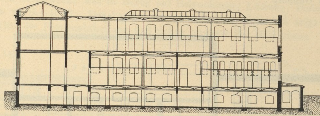
Längenschnitt.
