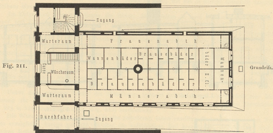
Volksbad an der Churfürstenstraße zu Mainz 224 ).
