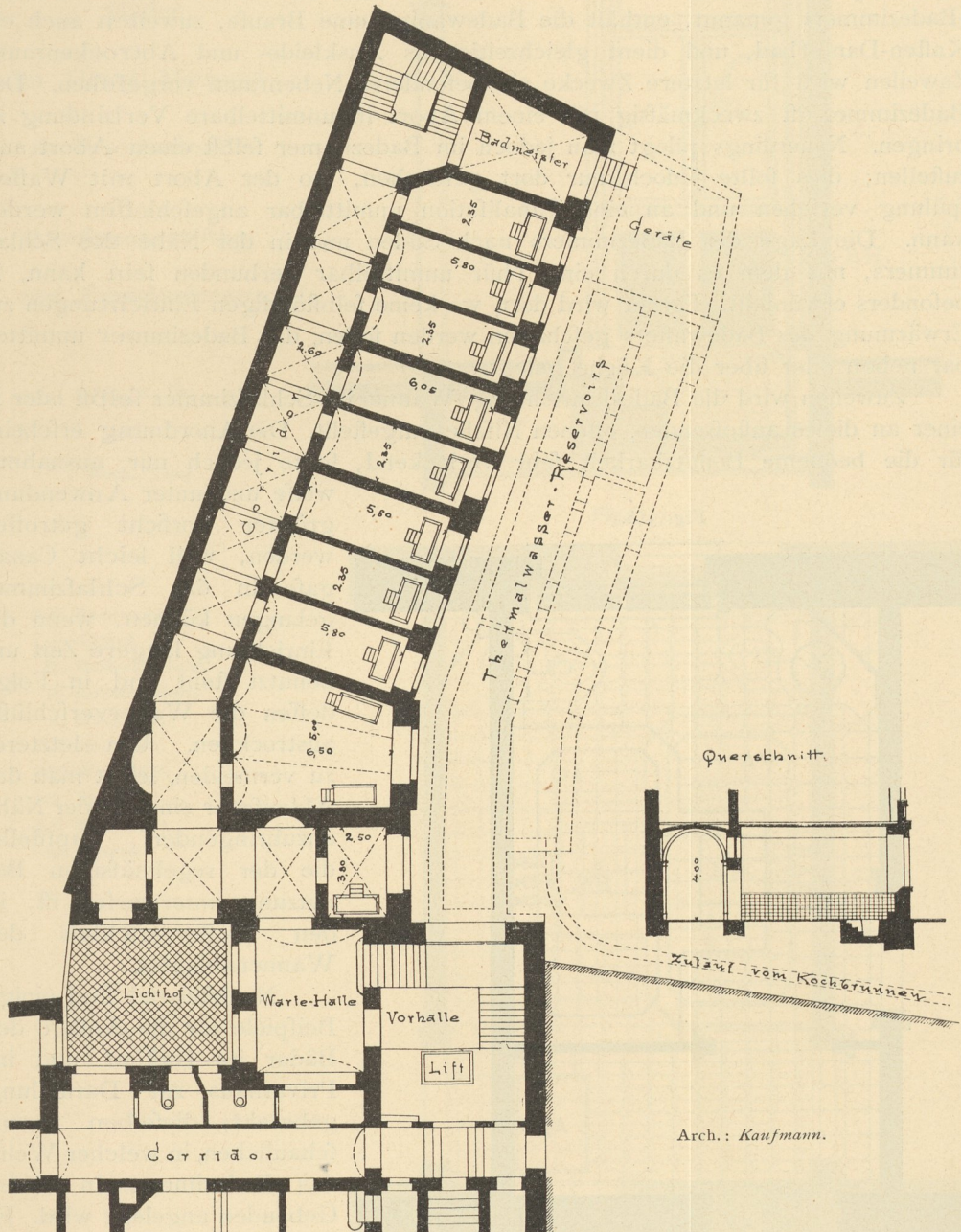
Süßwasser- und Thermalbäder mit Braufen im Gasthof »Zur Rose« zu Wiesbaden 269 ).
