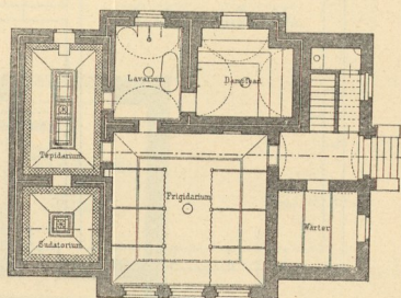
Grundriß.
