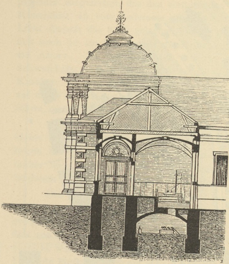
[Moorbad zu Bad Elfter. Querschnitt 250 ). — 1/250 n. Gr.
