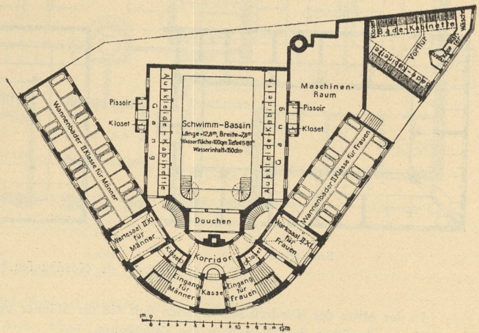
Erdgeschloß.
