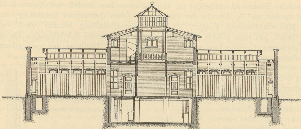
Längenschnitt.
