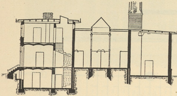
Längenschnitt.
