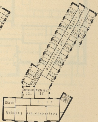
Obergechofs.
