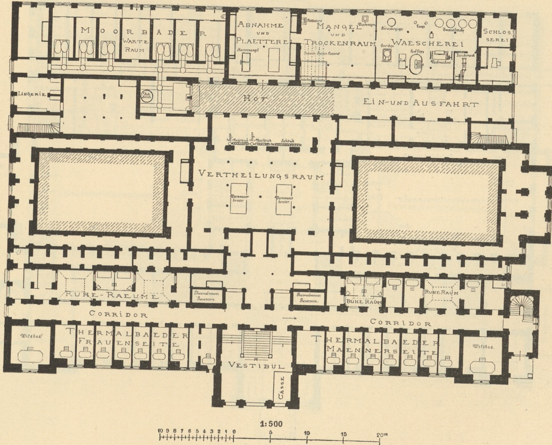
Augusta Victoria-Bad zu Wiesbaden. — Erdgeschoß 258) .
