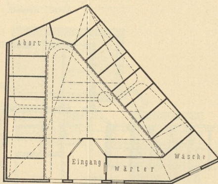
Grundriß. — 1/200 n. Gr. Volks-Brausebad zu Altona.
