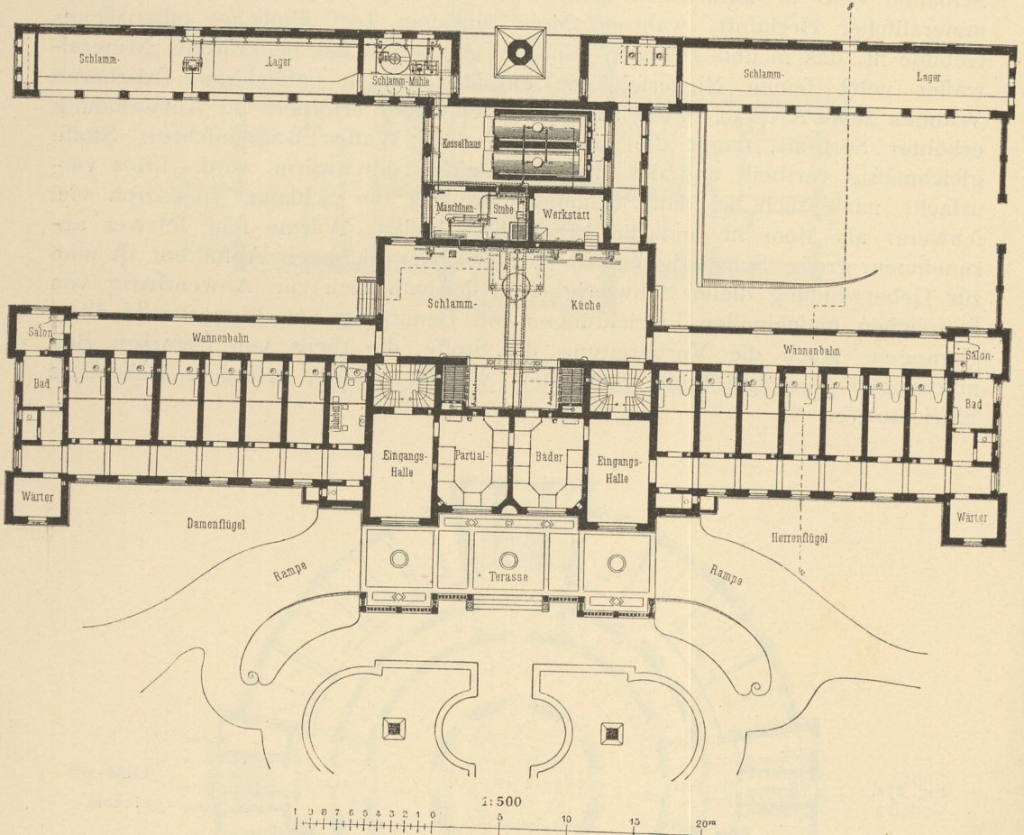
Schlamm- und Bade-Anstalt zu Nenndorf. — Erdgeschoss 248 .
