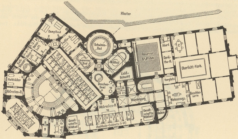
Obergeschoss.
