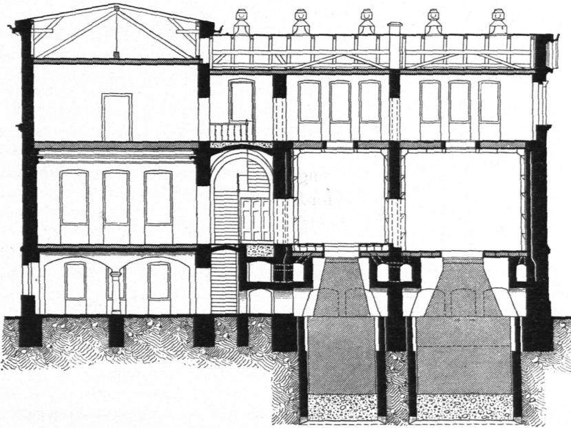
Längenschnitt.
