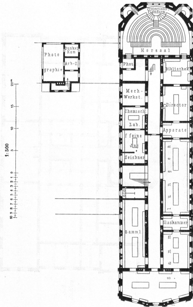
Obergeschofs.
