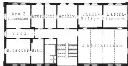
Obergeschofs.
