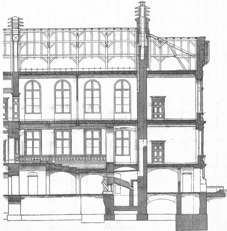
Längenschnitt.
