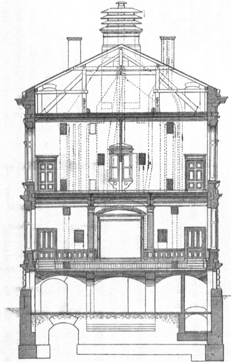
Querschnitt.
