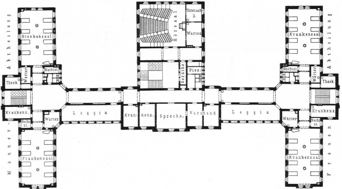
I. Obergechofs.
