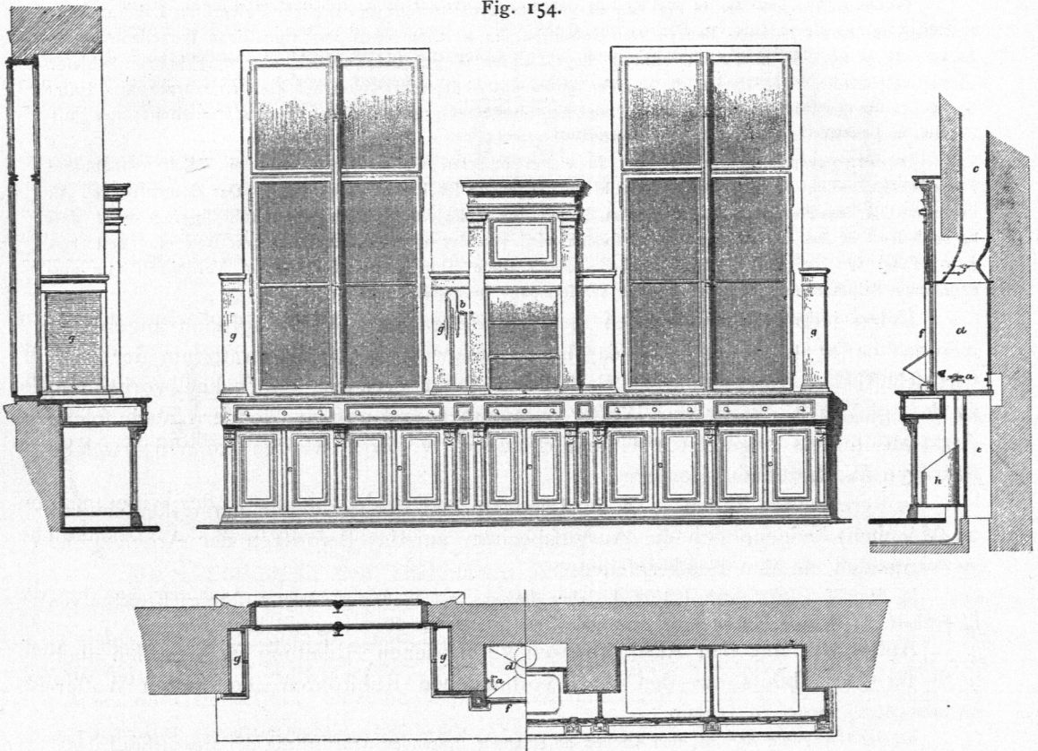
Arbeitsstische im chemischen Institut der Universität zu Budapest 159) .
