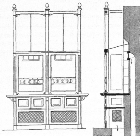
Abdampfschrank im chemischen Institut der Bergakademie zu Berlin 164 ). — 1/50 n. Gr.
