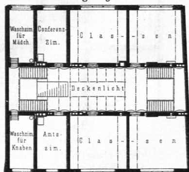
Doppelschule an der Niederwallstrasse zu Berlin. — \frac{1}{500} n. Gr.
