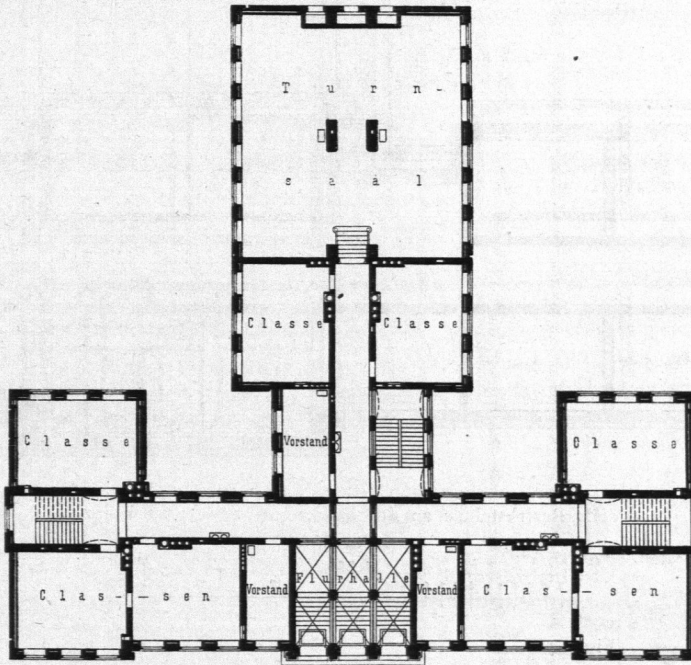
1:500 10 9 8 7 6 5 4 3 2 1 0 5 10 15 20 m Volksschule am Eppendorfer Weg zu Eimsbüttel bei Hamburg.
