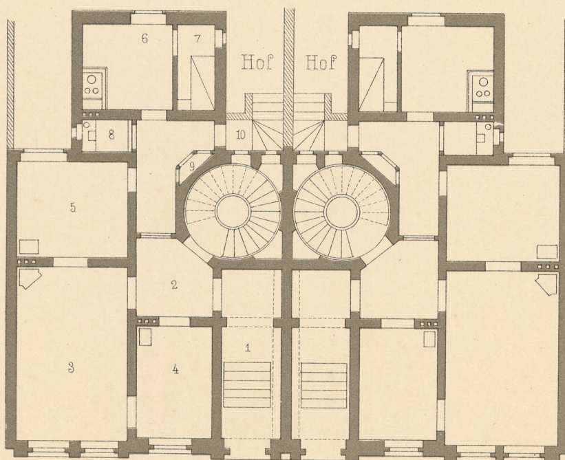
Erdgeschoss
