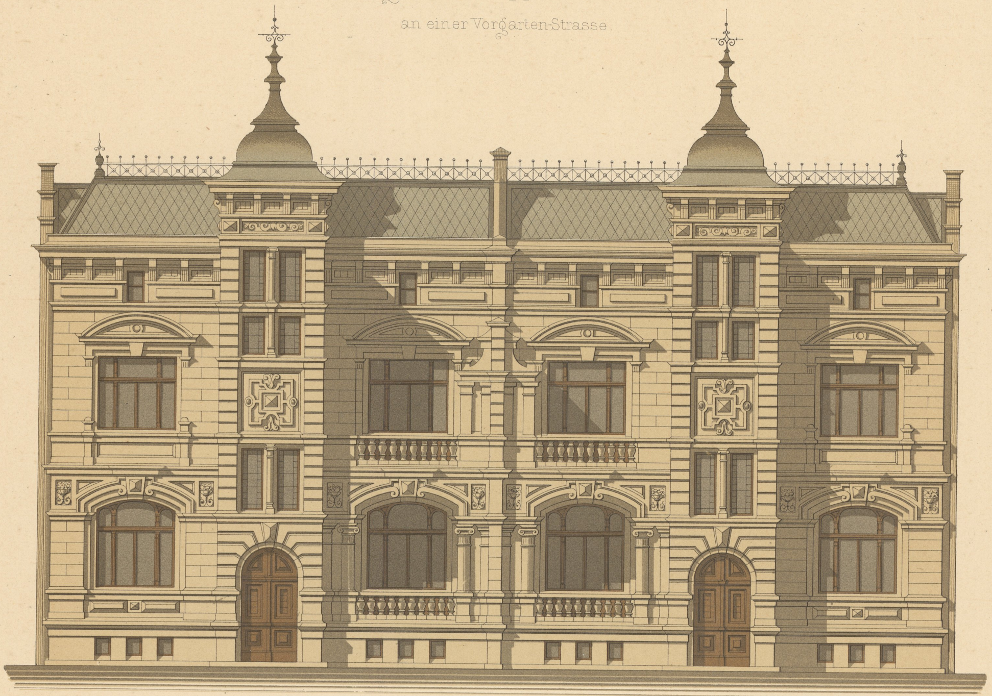
Anficht.
