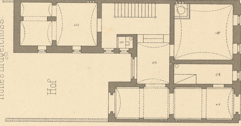
Kellergeschoss.
