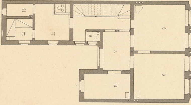
Hohes Erdgeschoss.
