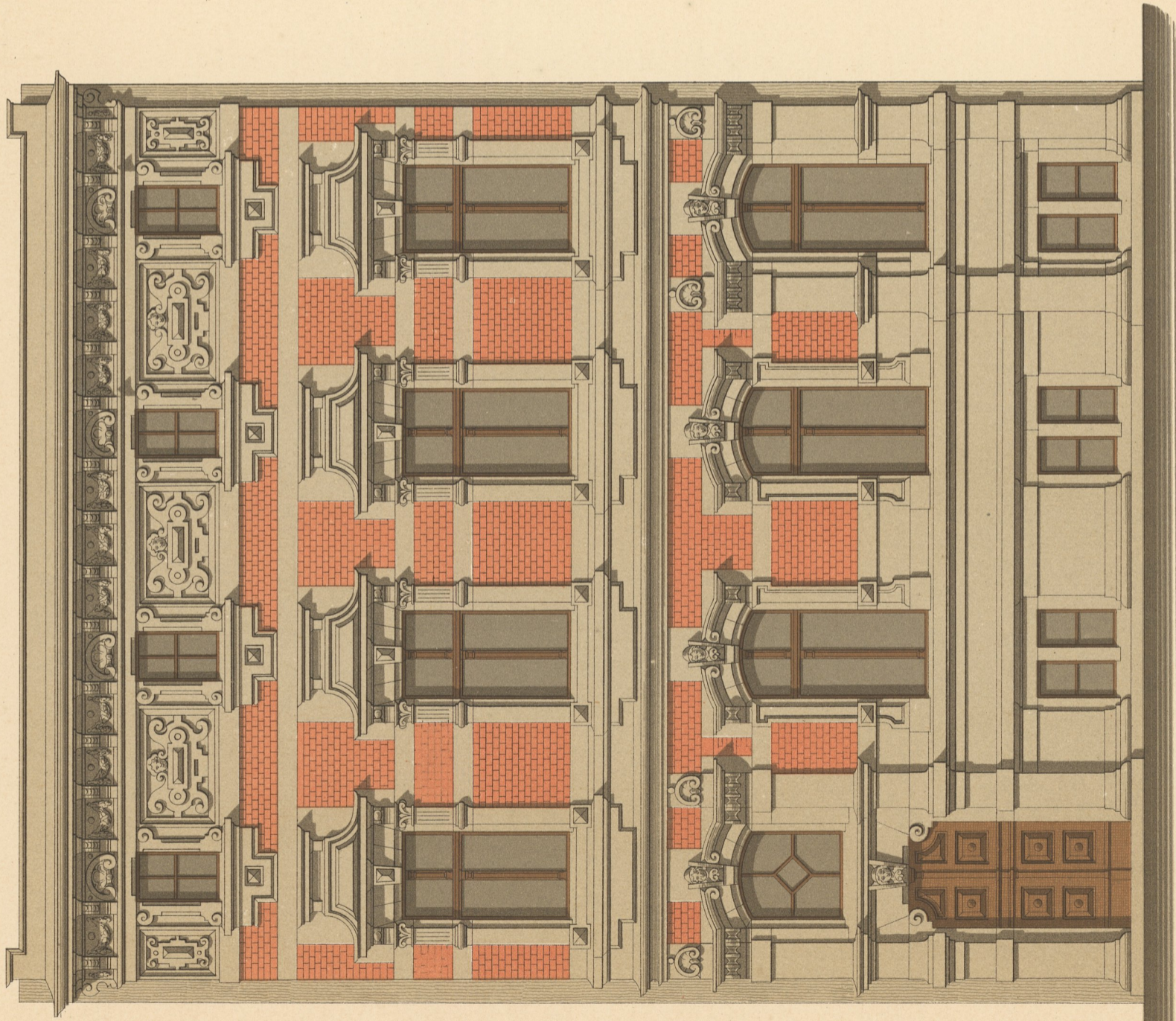
Anficht.
