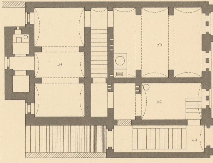
Kellergeschoss.
