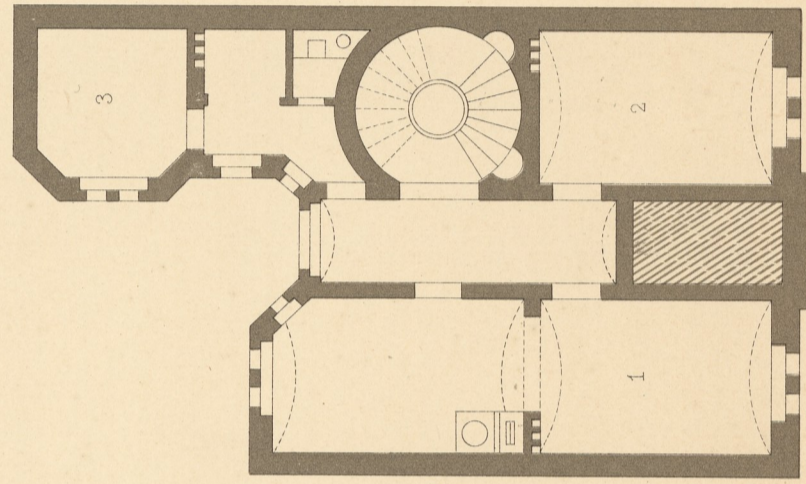
Kellergeschoss.
