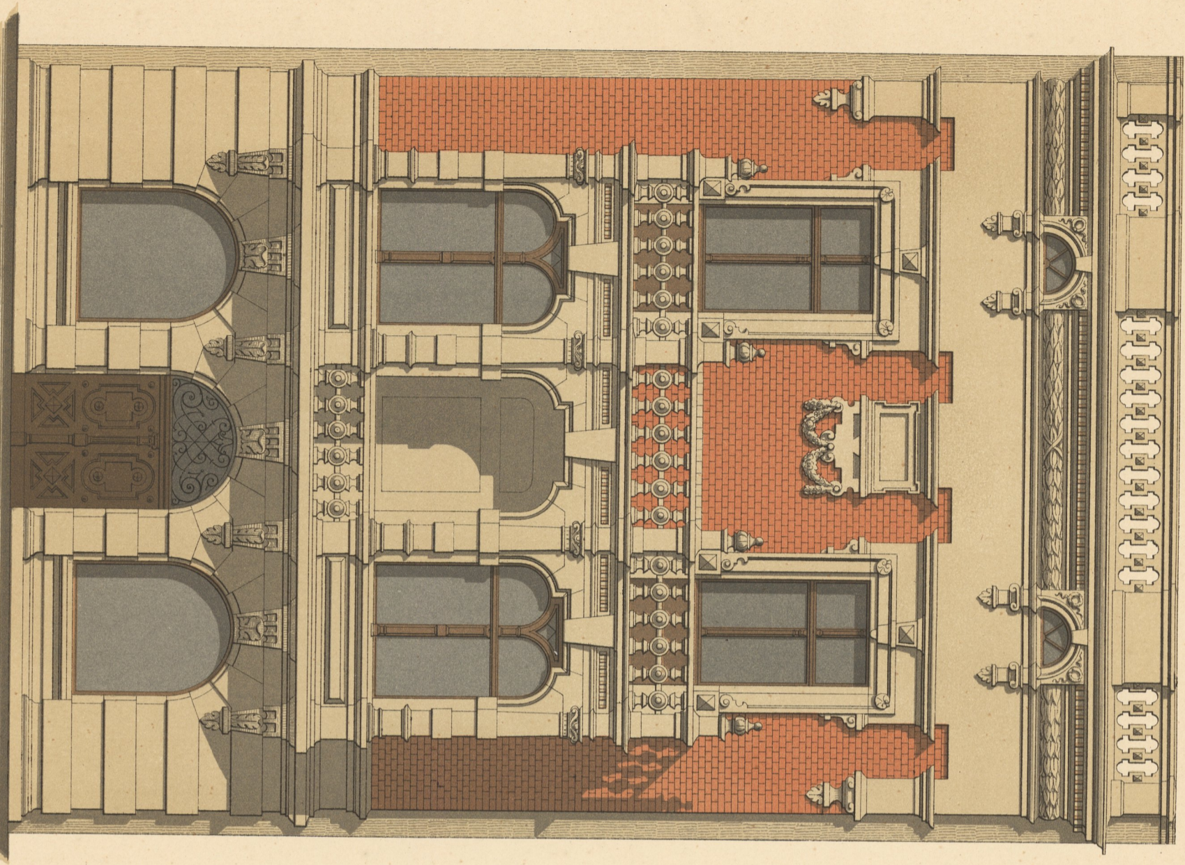
Anlicht.
