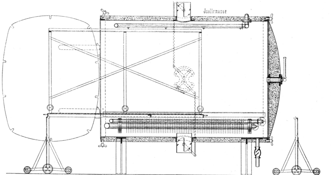
Längenschnitt.
