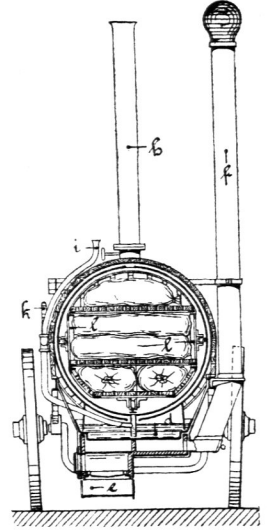
Querschnitt.
