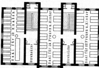
Städtisches Afyl für Obdachlose zu Elberfeld. — I. Obergeschofs.
