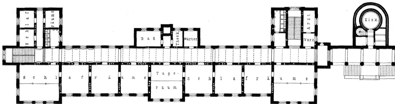
Siechenhaus. — Erdgefchofs.
