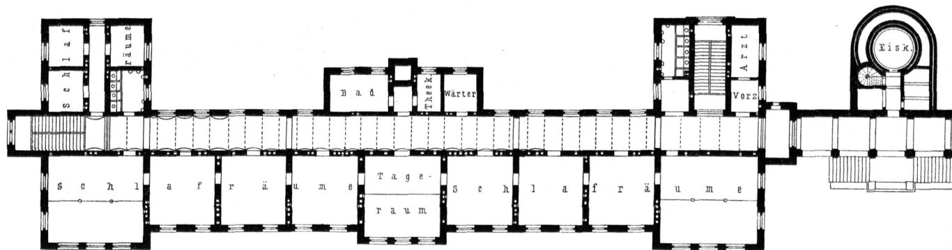
Siechenhaus. — Erdgefchofs.
