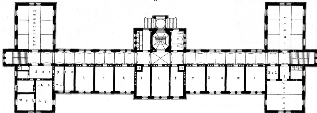
Seiten-Pavillon. — Erdgefchofs.
