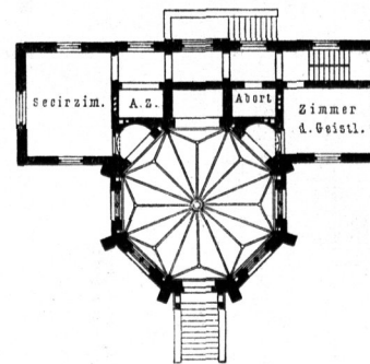
Leichenhaus. — Erdgefchofs.
