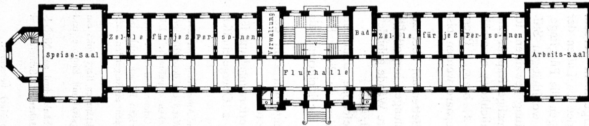
Fig. 95. Erdgeschoss.
