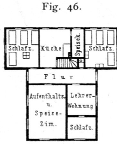
Ferienheim zu Büche. Erdgefchofs. Arch.: Held .
