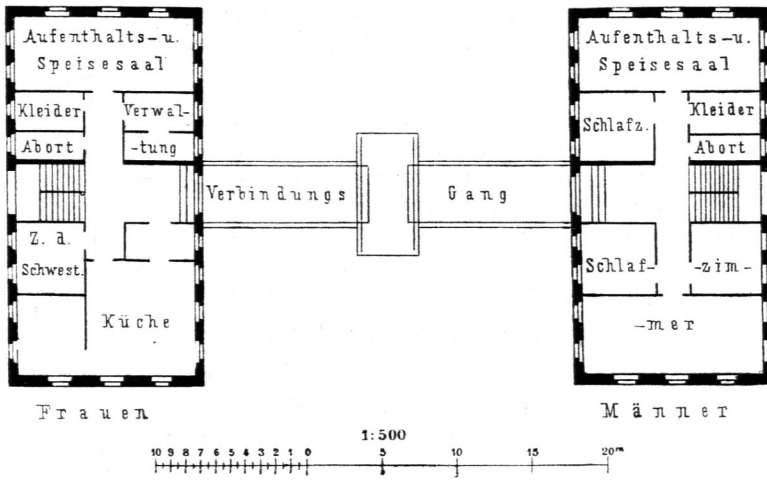
Hospizhaus »Lovifa« bei Straßburg. Erdgefchofs-Grundriß des Pflegehauses. Arch.: Perrin.
